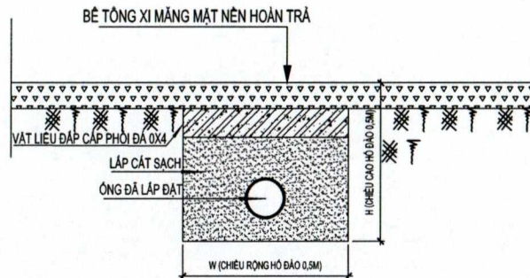
HOÀN TRẢ BỀ MẶT BÊ TÔNG MẶT ĐƯỜNG
