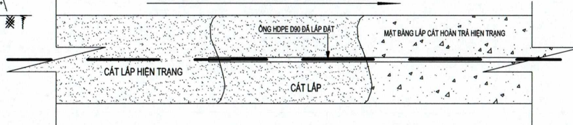
HƯỚNG THI CÔNG ĐƯỜNG ỐNG
