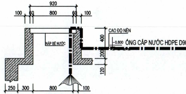
VỊ TRÍ CẤP VÀO BỂ CHỨA
