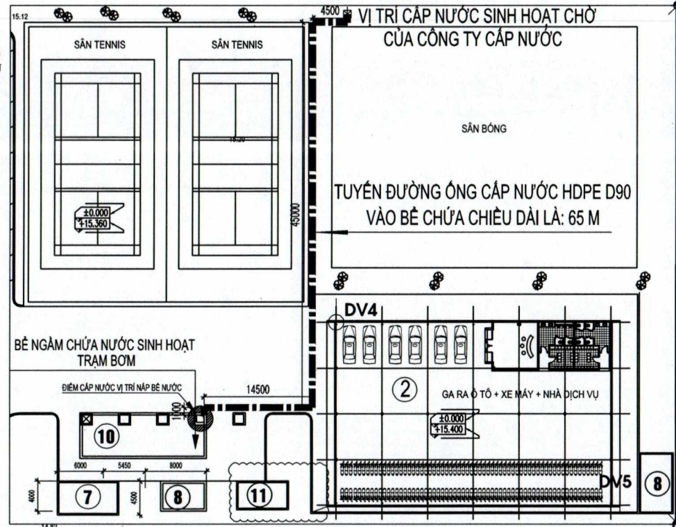
HƯỚNG THI CÔNG ĐƯỜNG ỐNG
