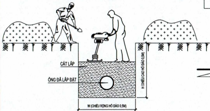
LẤP VÀ ĐÀM CÁT LÓT
